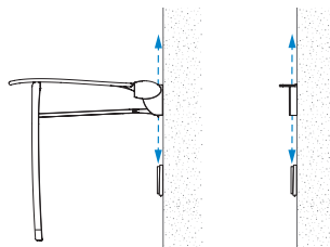
Gdy siedzisko nie jest używane, można je zastąpić półką 511921W
