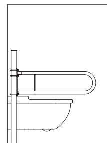
Przykład instalacji w WC
