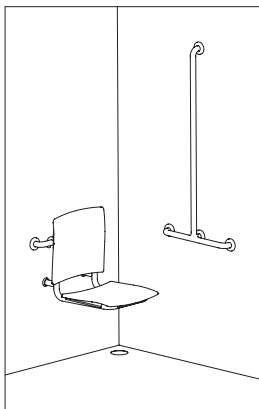
Przykład instalacji pod natryskiem
