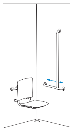
Możliwość regulacji miejsca pionowej poręczy
