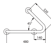
Model prawy - 5181D
