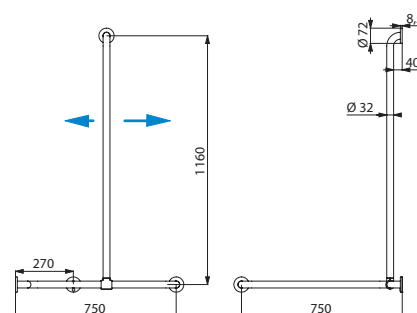
Możliwość regulacji w prawo lub w lewo pionowej poręczy
