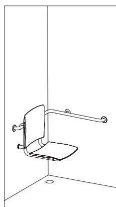
Przykład instalacji pod natryskiem
