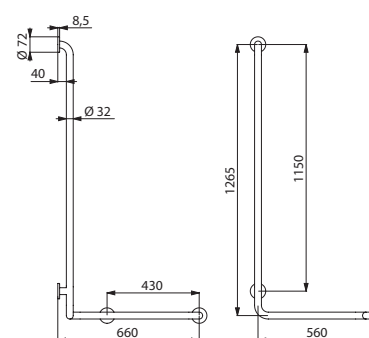
Model prawy - 5100DS
