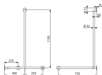
Model prawy - 5481D
