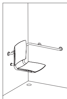
Przykład instalacji pod natryskiem
