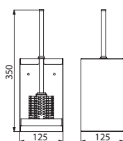
Pojemnik ze szczotką WC z wyciąganą podstawką
