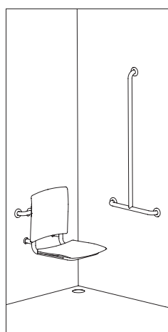
Przykład instalacji pod natryskiem
