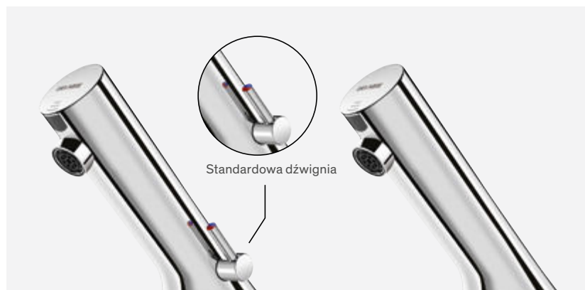
Zawór TEMPOMATIC 5 zasilanie sieciowe Nr DELABIE: 499000 - 449100
