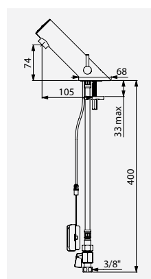
Bateria TEMPOMATIC 5 na baterie Nr DELABIE: 499006
