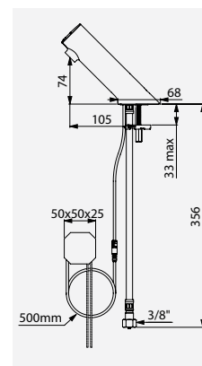
Zawór TEMPOMATIC 5 zasilanie sieciowe Nr DELABIE: 449100
