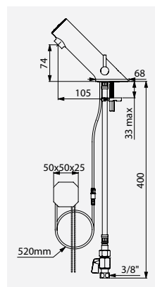
Bateria TEMPOMATIC 5 zasilanie sieciowe Nr DELABIE: 499000
