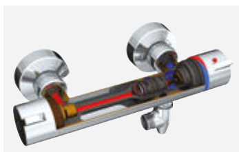
Przekrój H9768: niewielka ilość wody, izolacja termiczna i brak zaworów zwrotnych DELABIE: Przekrój3D_H9768 + 880
