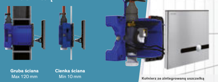
Kołnierz ze zintegrowaną uszczelką
