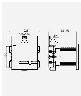
TEMPOMATIC z podwójnym uruchamianiem zasilanie sieciowe Nr DELABIE: 464SBOX-464000
