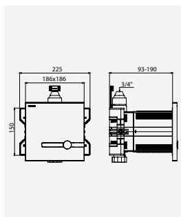
TEMPOMATIC z podwójnym uruchamianiem na baterie Nr DELABIE: 464PBOX-464006
