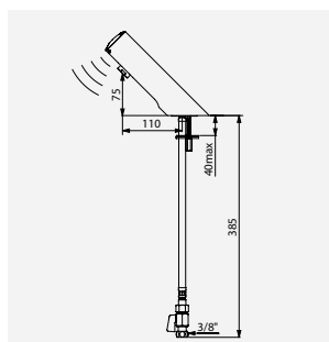
Zawór elektroniczny TEMPOMATIC 4 na baterie Nr DELABIE: 440006
