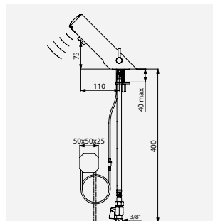
Bateria elektroniczna TEMPOMATIC MIX 4 zas. sieciowe Nr DELABIE: 490000
