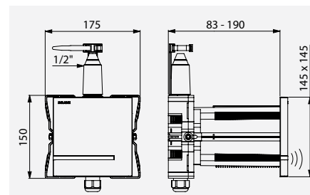
PODTYNKOWY ZAWÓR TEMPOMATIC 4 DO PISUARU Nr DELABIE: 430PBOX + 430006
