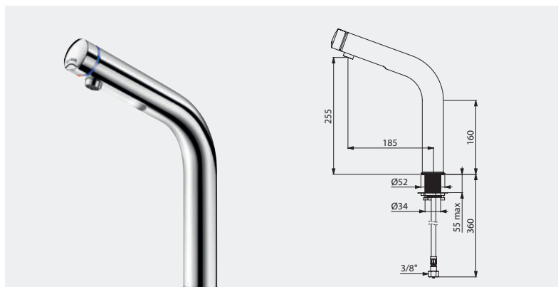
Czasowa bateria umywalkowa TEMPOMIX 3 H.250 mm Nr DELABIE: 794120
