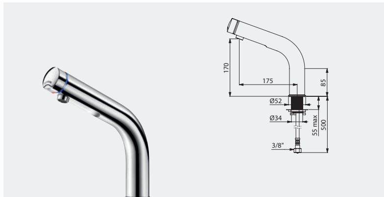
Czasowa bateria umywalkowa TEMPOMIX 3 H.170 mm Nr DELABIE: 794110
