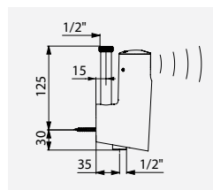
TEMPOMATIC 4, zawór liniowy Nr DELABIE: 479410
