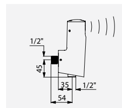
TEMPOMATIC 4, zawór kątowy Nr DELABIE: 479411
