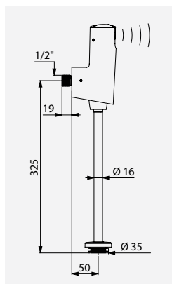
TEMPOMATIC 4, kompletny zestaw do standardowego pisuaru Nr DELABIE: 479412
