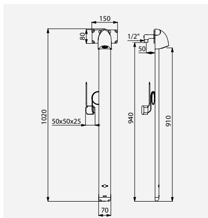
Elektroniczny panel SPORTING 2 SECURITHERM zasilanie sieciowe, podtylnkowe przyłącza wody Nr DELABIE: 714910
