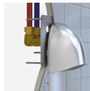
Podtylnkowe przyłącza wody od góry
