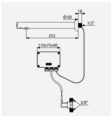
Długi model BINOPTIC Nr DELABIE: 379ENCL
