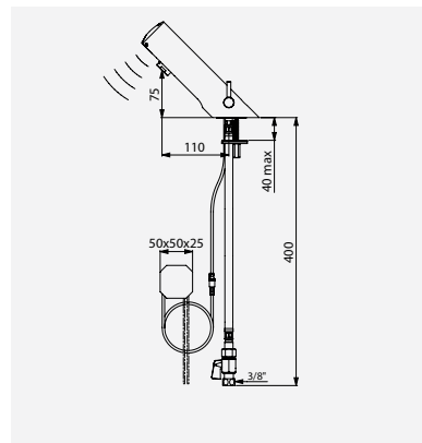
Bateria elektroniczna TEMPOMATIC 4 zasilanie sieciowe Nr DELABIE: 490000
