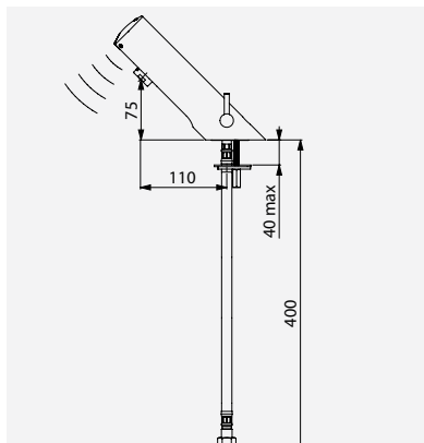
Bateria elektroniczna TEMPOMATIC 4 na baterie Nr DELABIE: 490006
