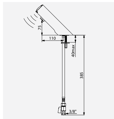
Zawór elektroniczny TEMPOMATIC 4 na baterie Nr DELABIE: 440006
