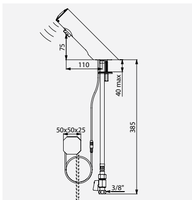
Zawór elektroniczny TEMPOMATIC 4 zasilanie sieciowe Nr DELABIE: 440000
